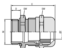
SKINTOP® MS-M
