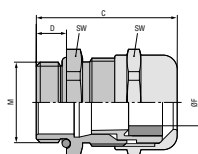
SKINTOP® MSR-M
