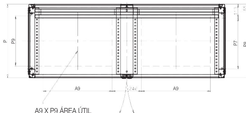
SECCIÓN B-B
