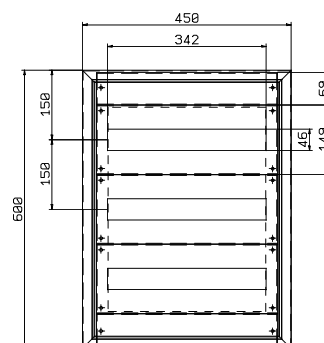
CLNMOD4560 57 MÓDULOS
