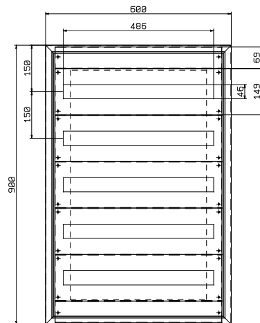
CLNMOD6090 135 MÓDULOS
