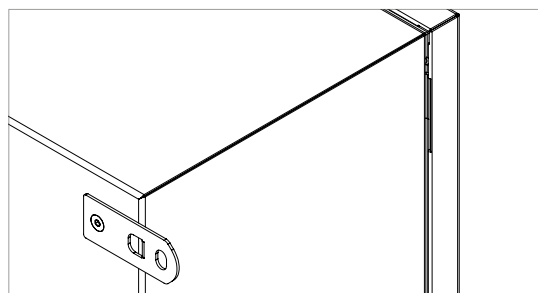
DETALLE POSTERIOR CAJAS CON ESTRIBO HORIZONTAL
