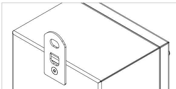
DETALLE POSTERIOR CAJAS CON ESTRIBO
