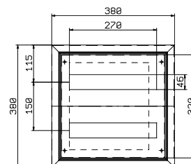
CLNMOD3838 30 MÓDULOS
