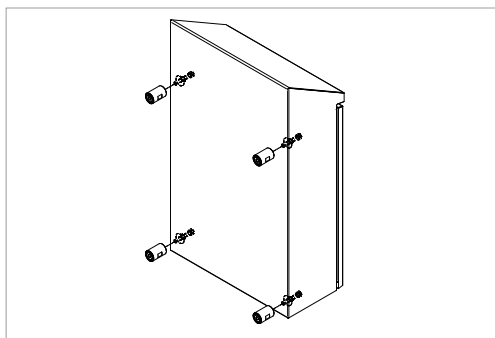
DETALLE DE FIJACIÓN TRASERA CON TORNILLO CORTO
