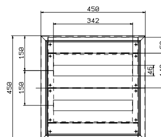
CLNMOD4545 38 MÓDULOS
