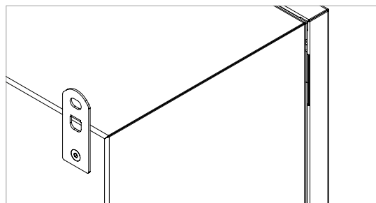
DETALLE POSTERIOR CAJAS CON ESTRIBO VERTICAL
