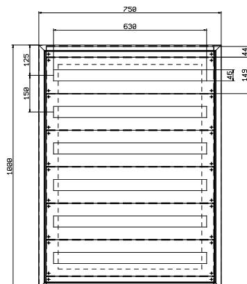
CLNMOD75100 210 MÓDULOS
