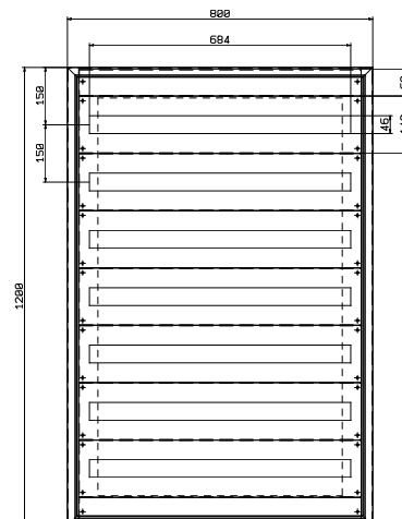
CLNMOD80120 266 MÓDULOS
