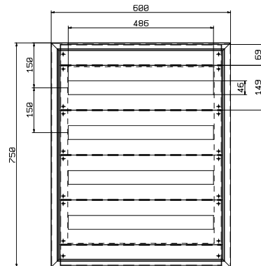
CLNMOD6075 108 MÓDULOS
