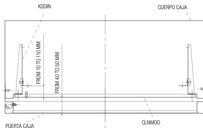
VISTA SECCIÓN CAJA CON ACCESORIOS
