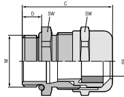
SKINTOP® MSR-M
