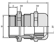
SKINTOP® MS-M
